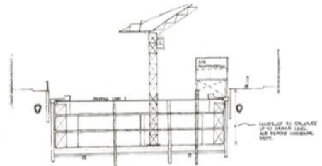
SECTION A-A (1:200)
