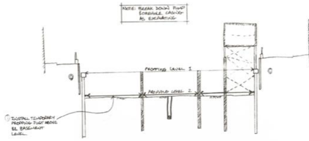
SECTION A-A (1:200)
