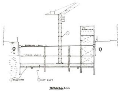
SECTION A-A (1:200)
